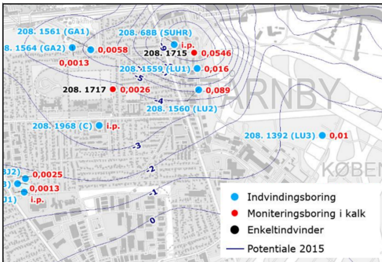
Figur 3: Sum af PFAS-stoffer i µg/l i området ved Tårnby Forsynings kildepladser. Årsrapport, Tårnby Forsyning 2022 .
