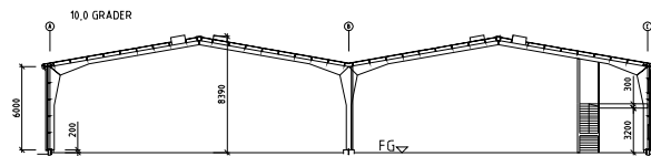
SEKTION A-A
